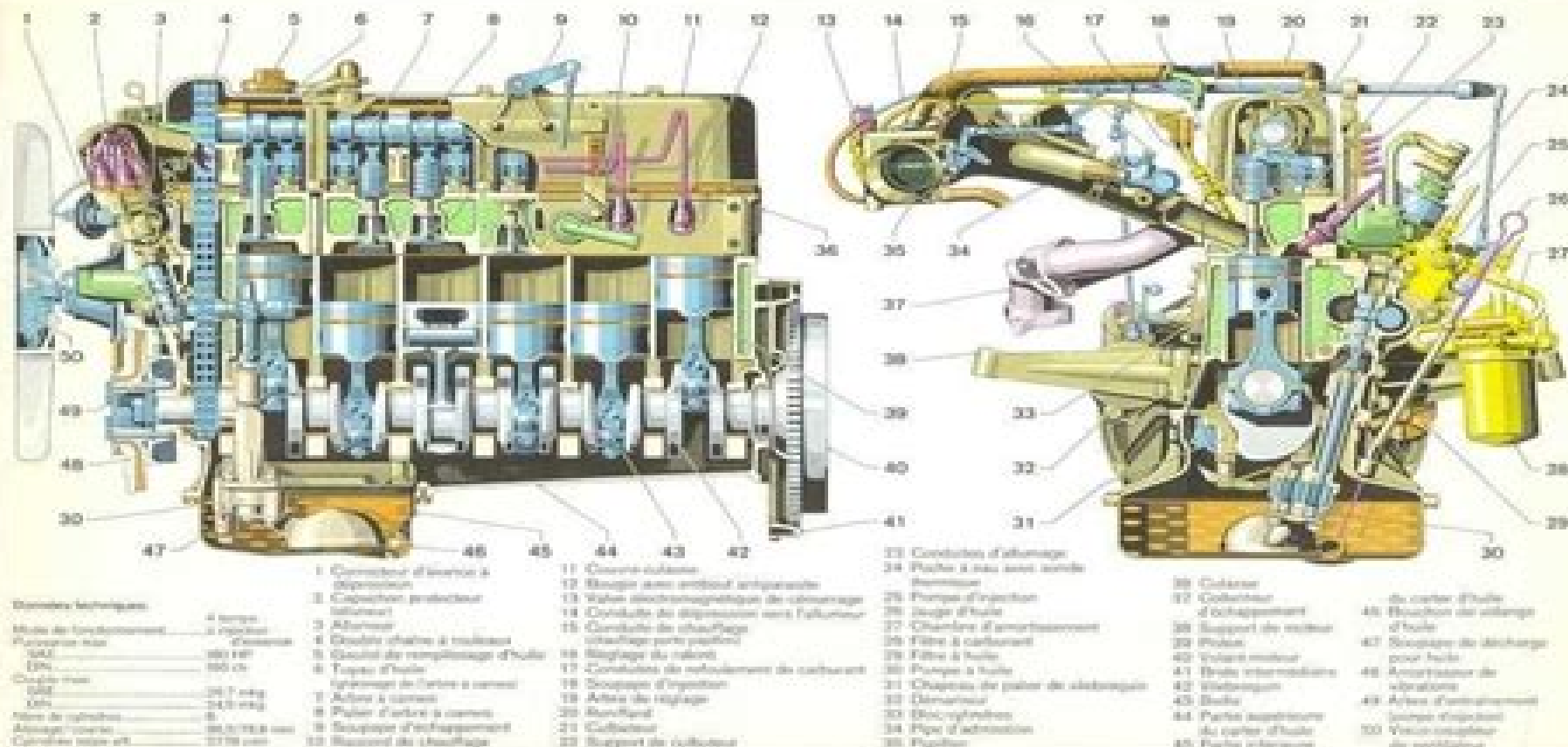
Moteur M 130 Coupes longitudinale et transversale Type 260 SE
