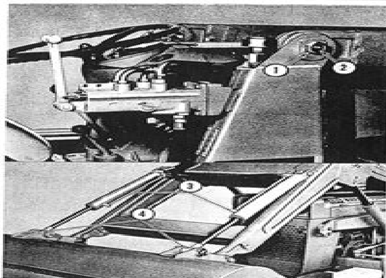
Fig. 12 - Lubrication Points
