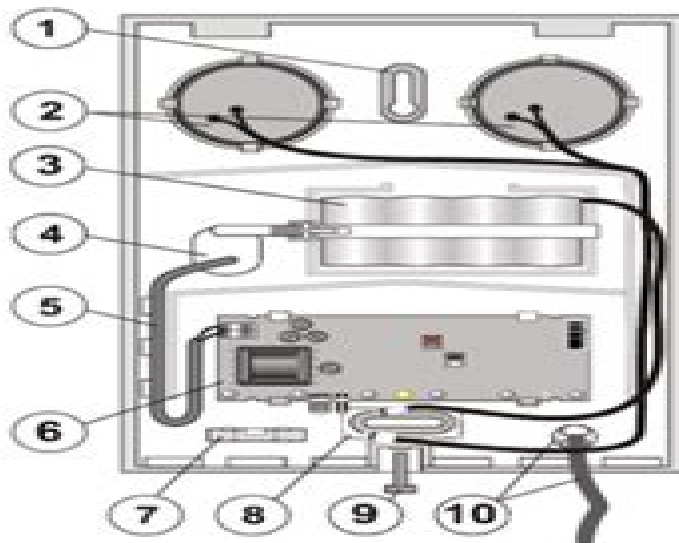
Figura: 1 - agujero de montaje; 2 - transformadores electroacústicos; 3 - acumulador NiCd; 4 - agujero para conductor al cable; 5 - cable de alimentación; 6 - piezas de electrónica de la sirena; 7 - nivel de agua integrado; 8 - agujero de montaje con detección de tiro; 9 - tornillo de la tapa de la sirena; 10 - cuerda con pasador que permite suspender la tapa de la sirena (se puede separar fácilmente apretando el campo)
