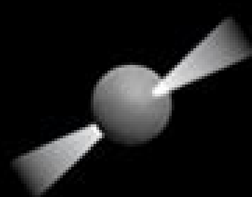
pulsars
