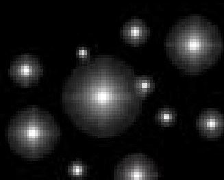
amas stellaires
