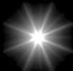
quasars
