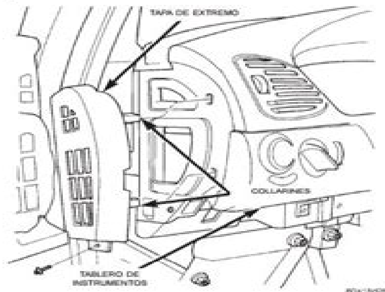
Fig. 34 Tapa de extremo izquierdo del tablero de instrumentos
