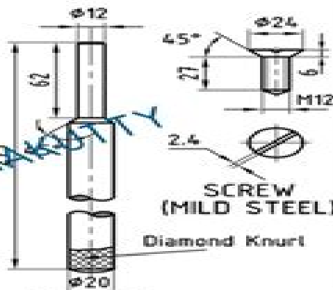
TOMMY BAR (MILD STEEL)
