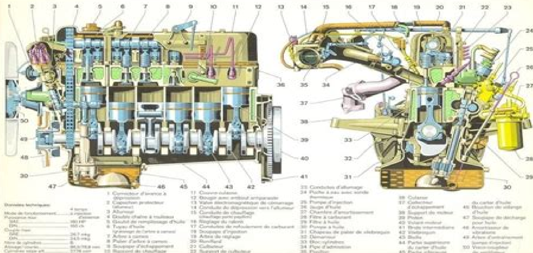
Moteur M 130 Coupes longitudinale et transversale Type 280 SE
