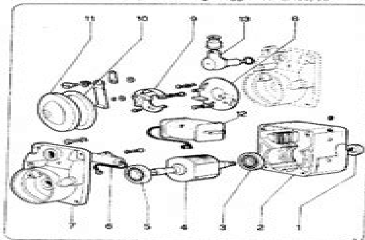
Fig. 16 - Particolari magnete
