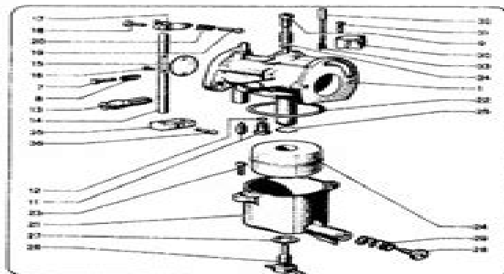
Fig. 14 - Particolari carburatore Serie LA 65-80
