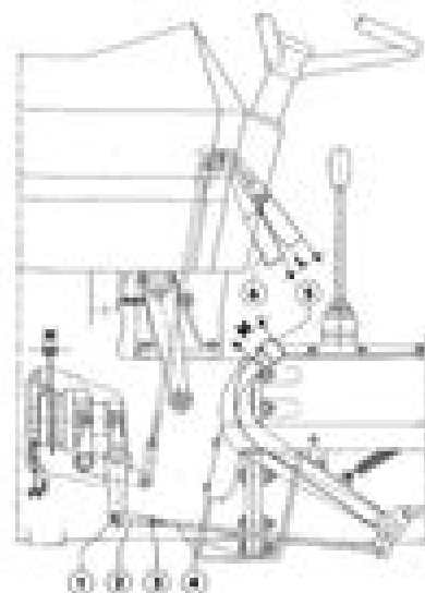
Fig. 7 - Registrazione organi di comando di frizione presso di potenza e frizione presso di potenza.
