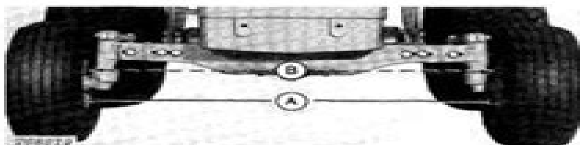
Fig. 31—Checking Toe-In
