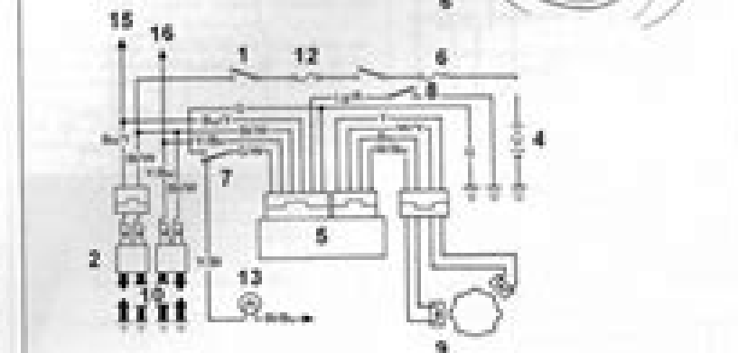
Circuito de principio de encendido e implantación de sus diferentes componentes:
