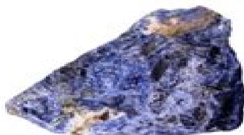
Sodalite
