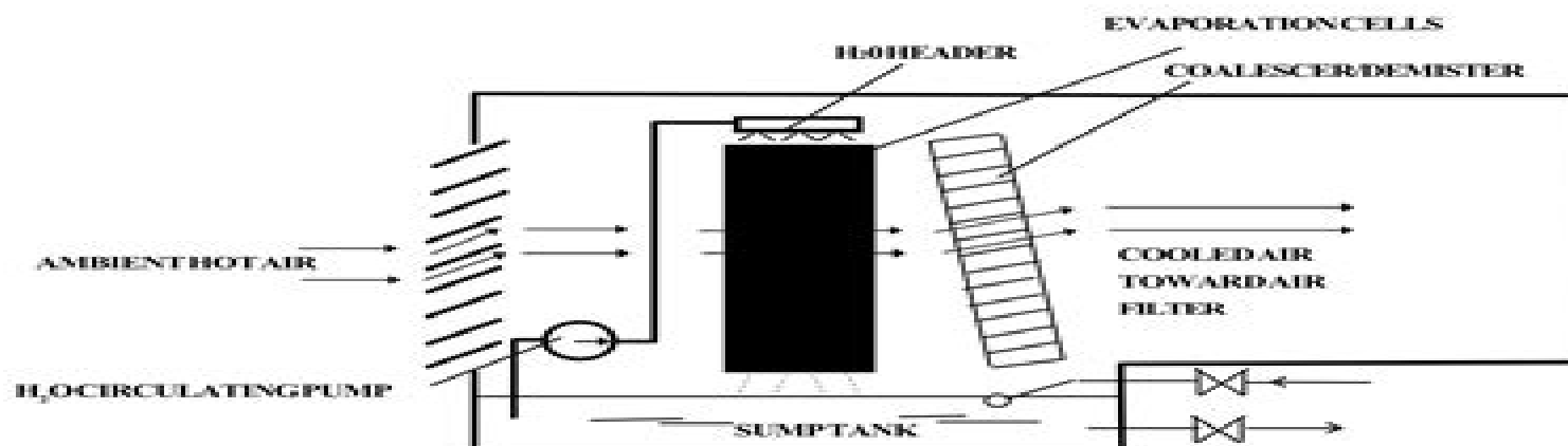
Fig. Th.14 Evaporative cooler
