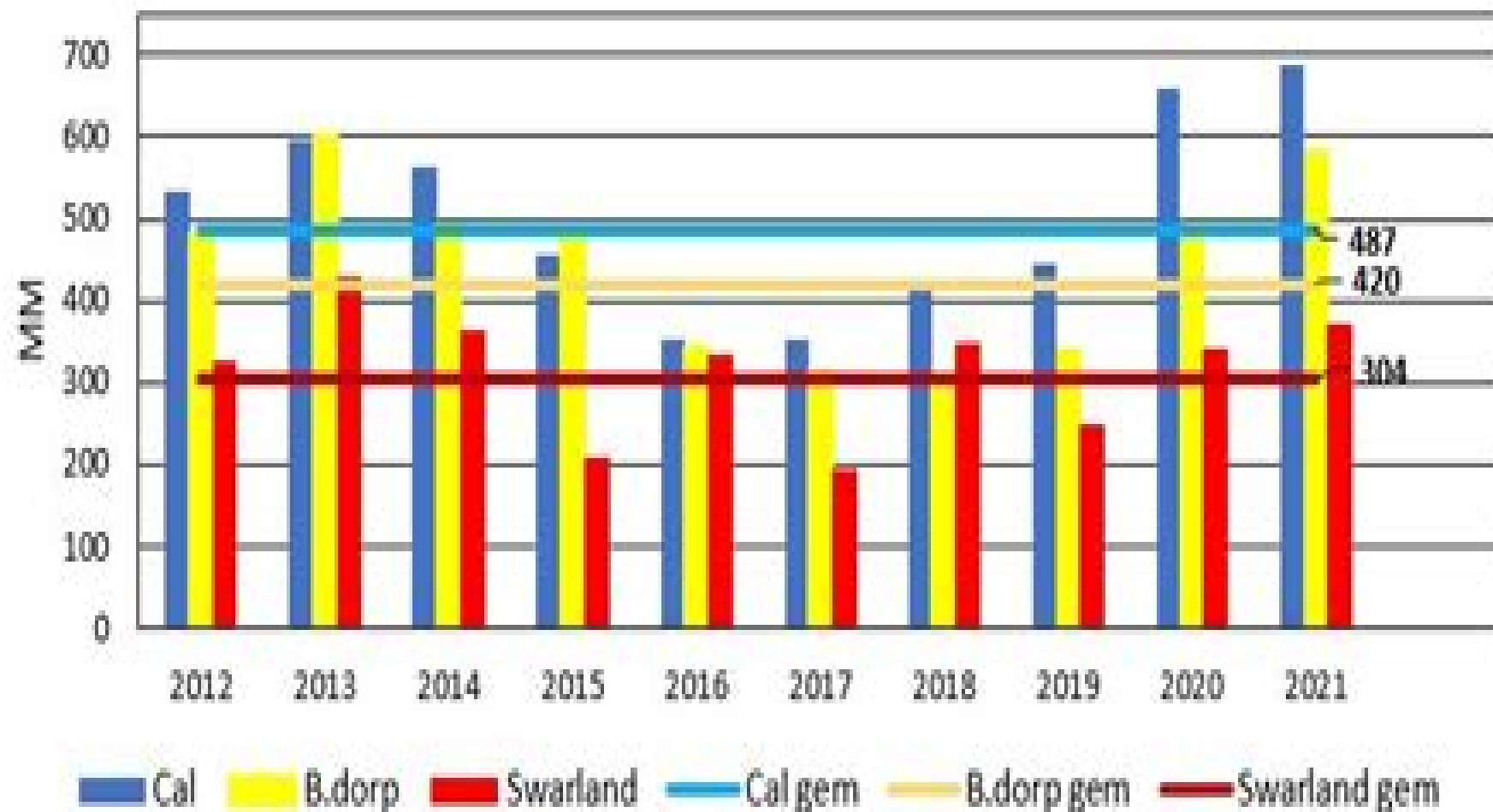
Figuur 1: Caledon-, Bredasdorp- en Swartland-area gemiddelde jaarlikse reënval
