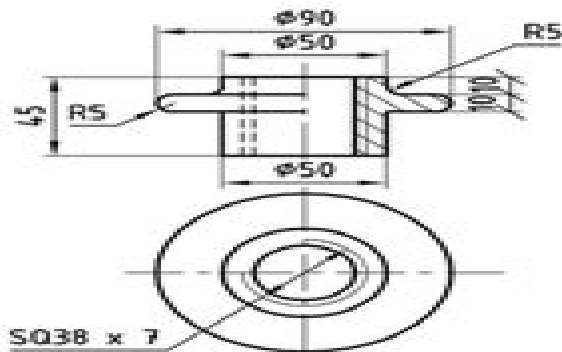
NUT (GUN METAL)
