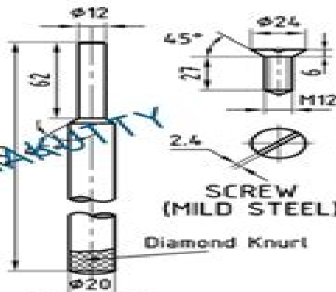
TOMMY BAR (MILD STEEL)
