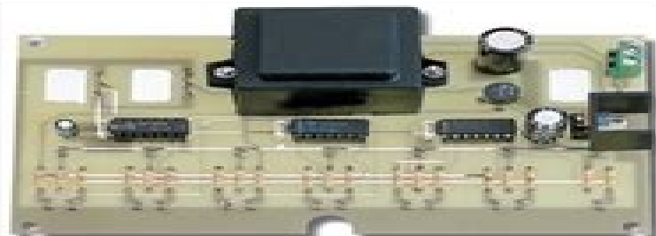
Figure 600 : Avant de souder les LED sur le circuit imprimé, vous devez, si vous avez décidé de monter la table de vérité électronique dans son boîtier, mettre en place 4 entretoises et la face avant (voir texte).
