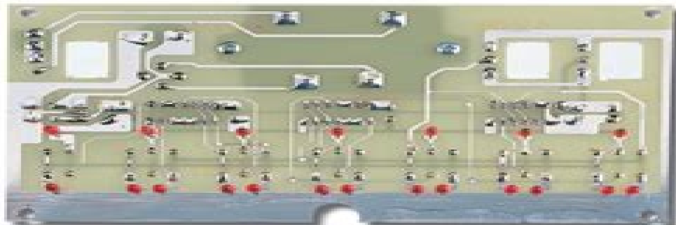
Figure 601 : Une fois le montage terminé, vous pouvez fixer le circuit imprimé à l'intérieur de son boîtier plastique.
