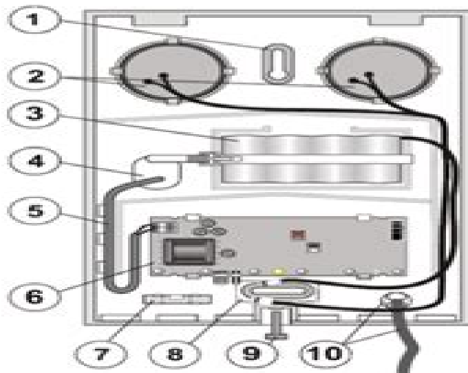
Figura: 1 - agujero de montaje; 2 - transformadores electroacústicos; 3 - acumulador NiCd; 4 - agujero para conducir el cable; 5 - cable de alimentación; 6 - piezas de electrónica de la sirena; 7 - nivel de agua integrado; 8 - agujero de montaje con detección de tiro; 9 - tornillo de la tapa de la sirena; 10 - cuerda con pasador que permite suspender la tapa de la sirena (se puede separar fácilmente apretando el campo).
