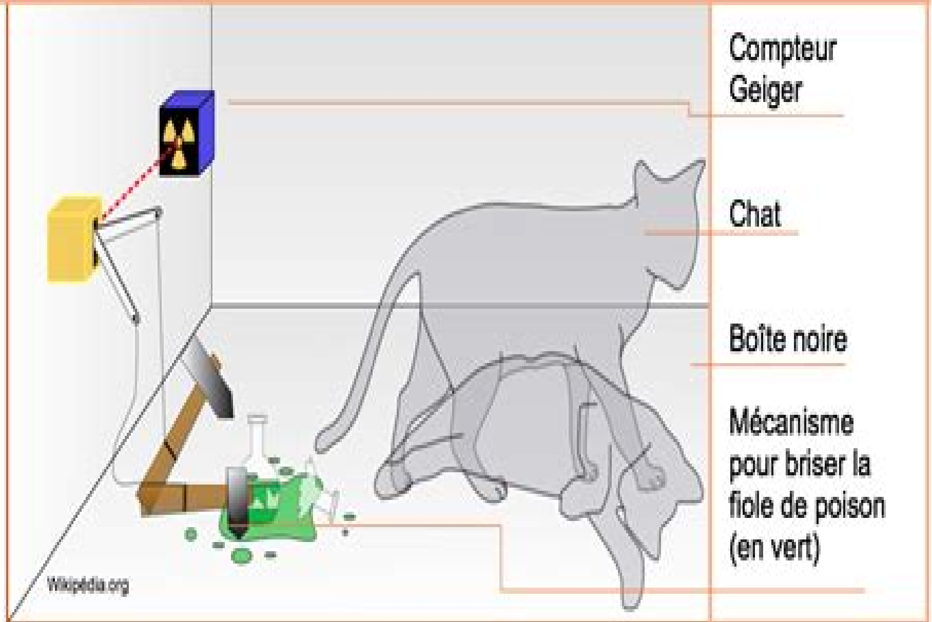
Fig. 2 : l'expérience du « chat de Schrödinger »
