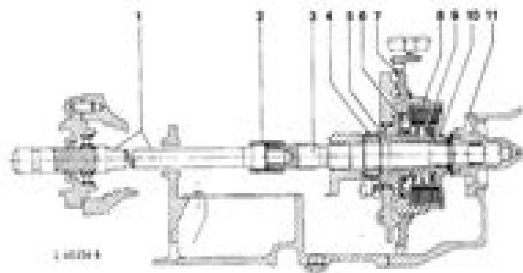
Bild 1 - Verschiebbare, stufenlose Zapfenwelle 140 U/min - Schnitt
