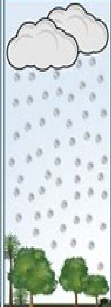
Graupel
