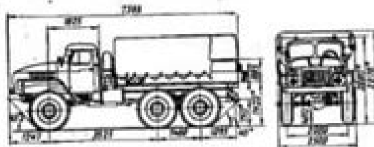
Рис. 1.3. Габариты и конструктивные размеры стандартных типов
