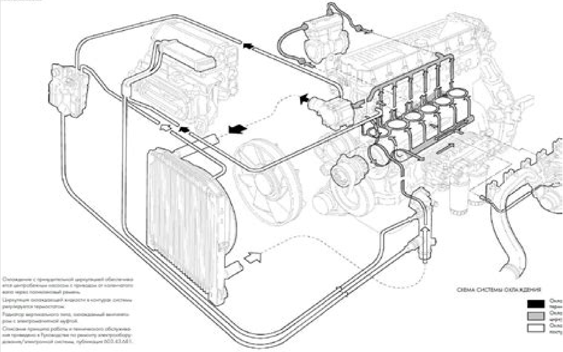
5432 СИСТЕМА ОХЛАЖДЕНИЯ Рисунок 214
