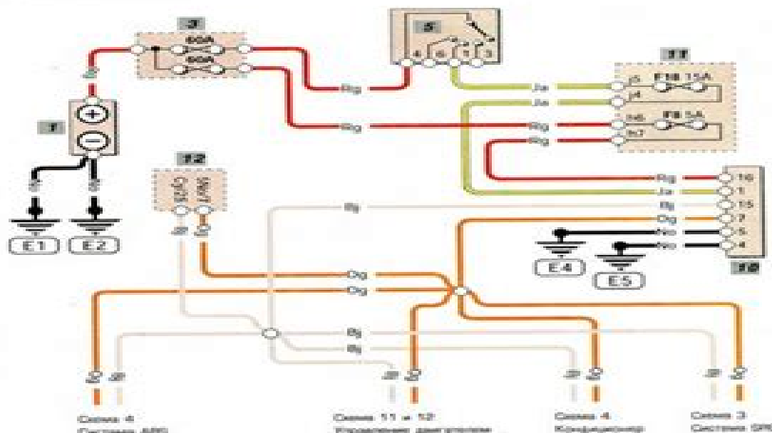
Диагностический разъем
