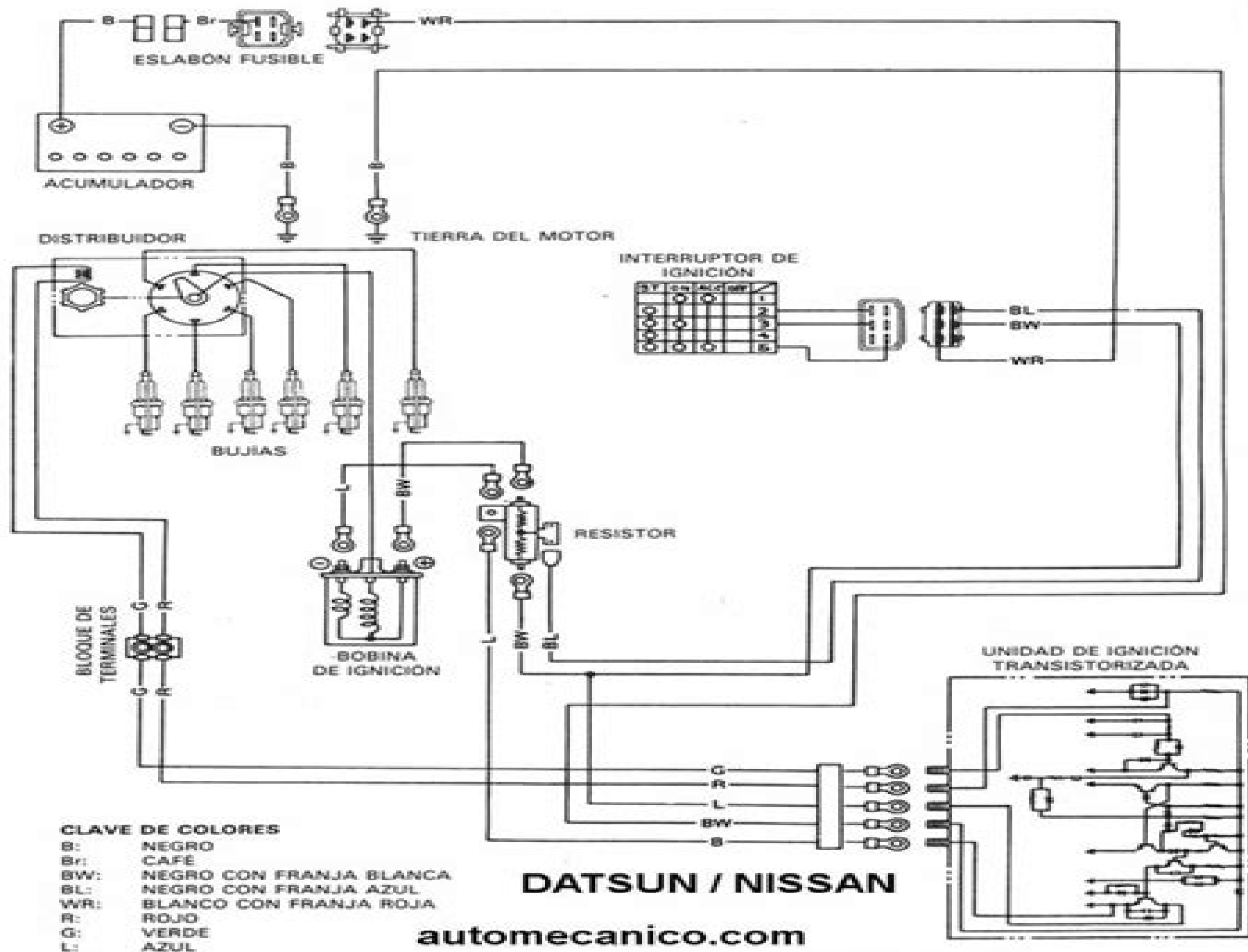
Diagrama del encendido electrónico, modelos 1975-1978 de seis cilindros
