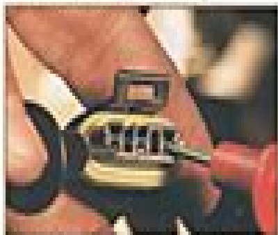
Fig. 3.2. Exemplo de verificação de curto-circuito no chicote do sensor VSS (entre os bornes 1 e 3 do terminal elétrico do sensor).
