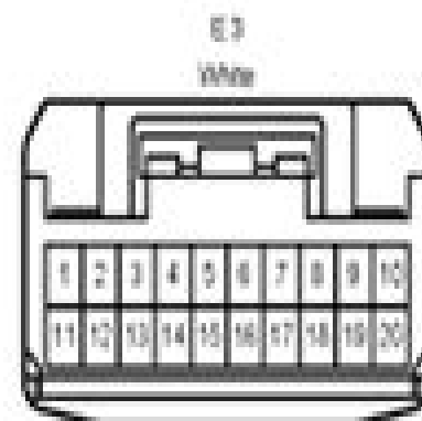
E3 Connector
