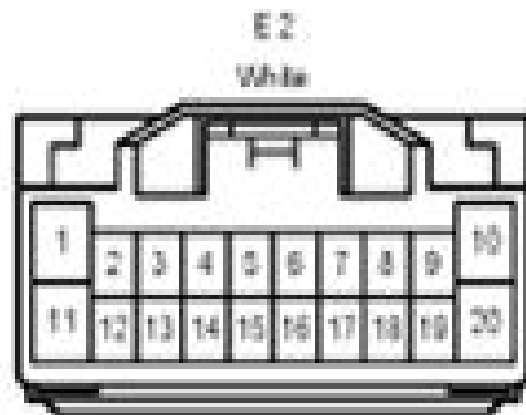
E2 Connector
