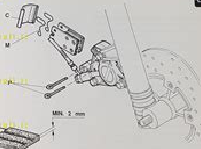
Fig. 23 (rimozione pastiglie)
